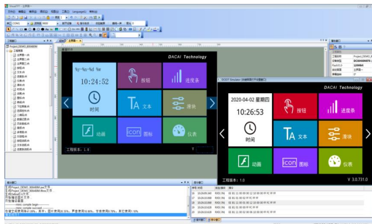
图 9-1 VisualTFT 主界面
