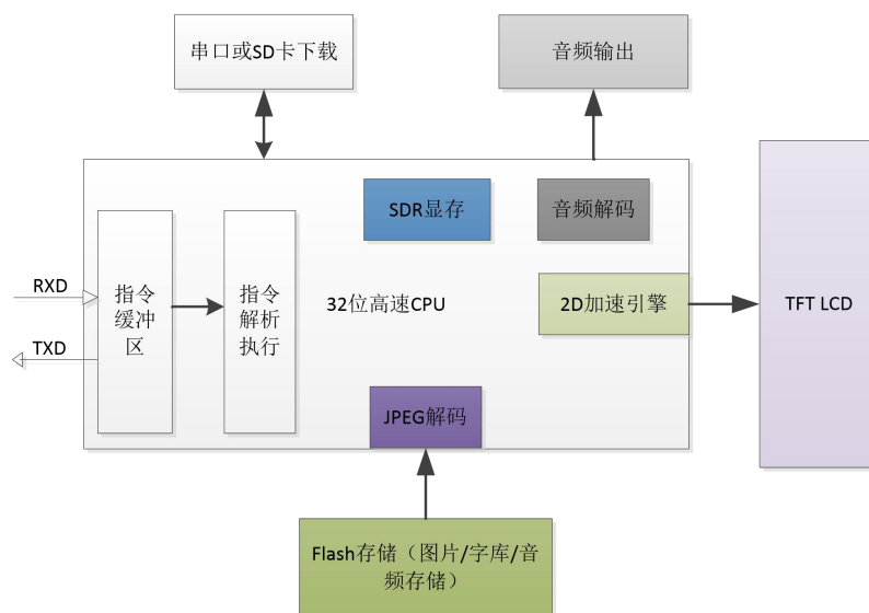
图 3-1 M 系列串口屏内部结构图
